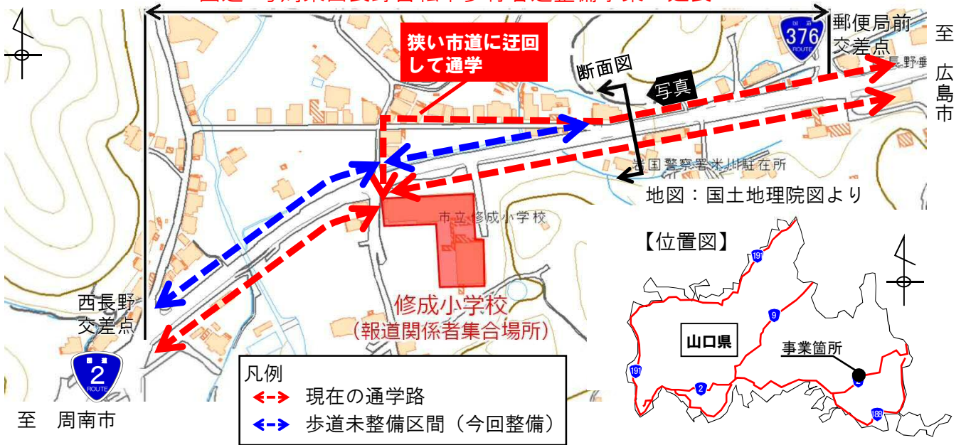
国道2号周東西長野自転車歩行者道整備事業 延長600m
