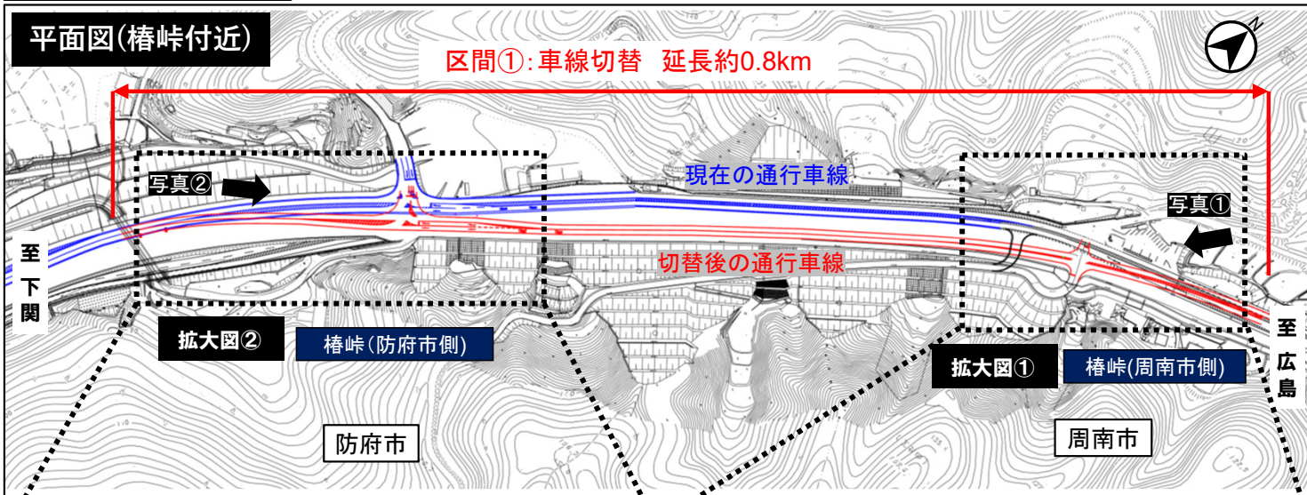
拡大図② [現在] (樺峠 防府市側付近)
