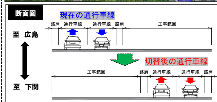
断面図
