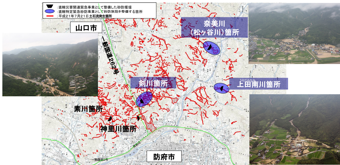
21 図 2.2.4 砂防事業実施箇所
